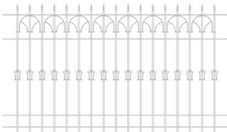
Zaunfeld Fl. 25x8 mm, Vkt. 14 mm
