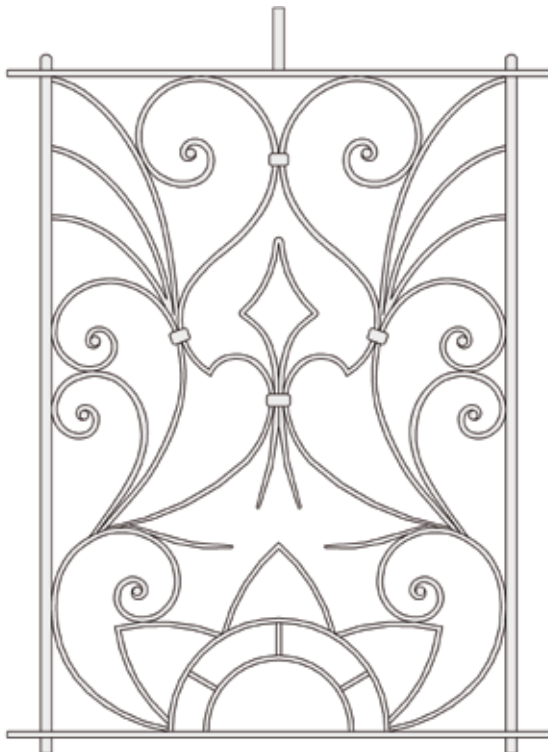
Mittelstück Vkt. 14 mm Fl. 14x6 mm
