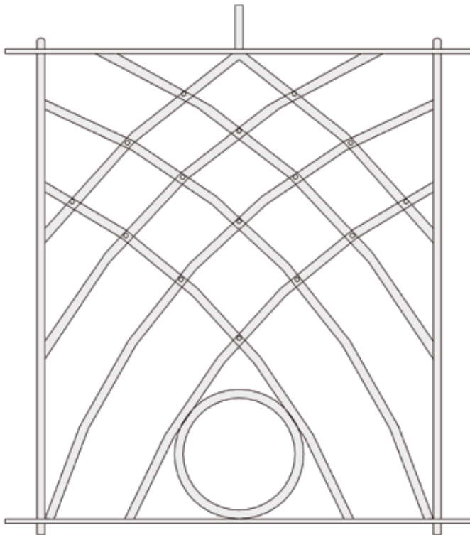
Mittelstück Vkt. 14 mm Fl. 16x6 mm
