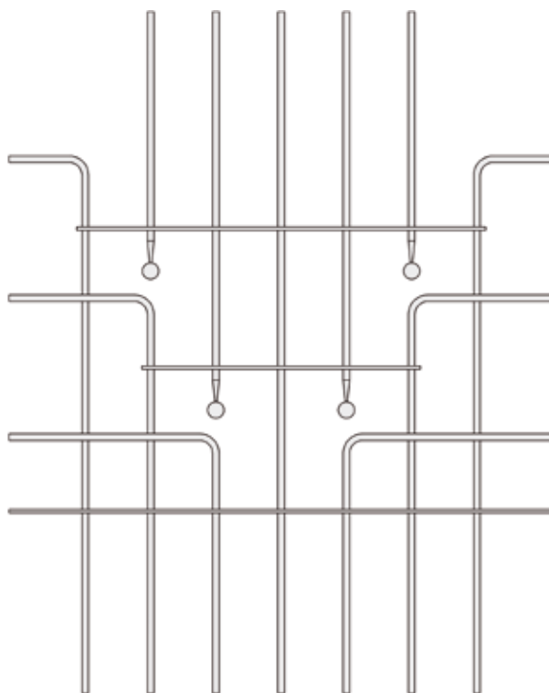
Türfüllung Fl. 30x6 mm, Rund 12 mm
