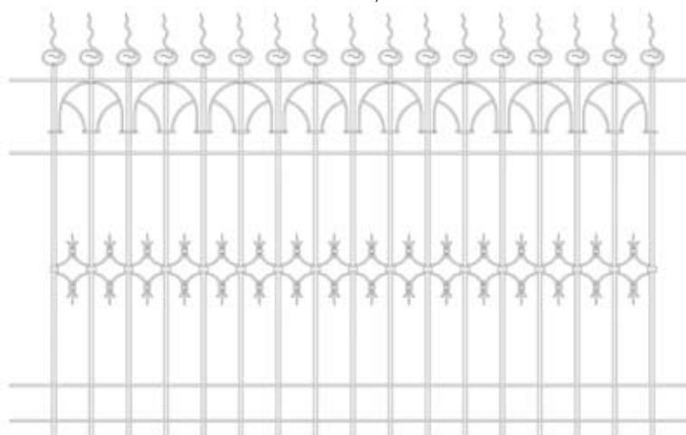
Zaunfeld Fl. 25x8 mm, Vkt. 14 mm
