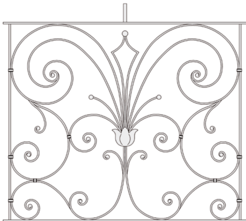
Mittelstück Vkt. 14 mm Fl. 14x6 mm
