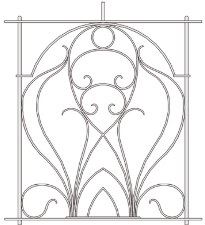
Mittelstück Vkt. 14 mm Fl. 14x6 mm
